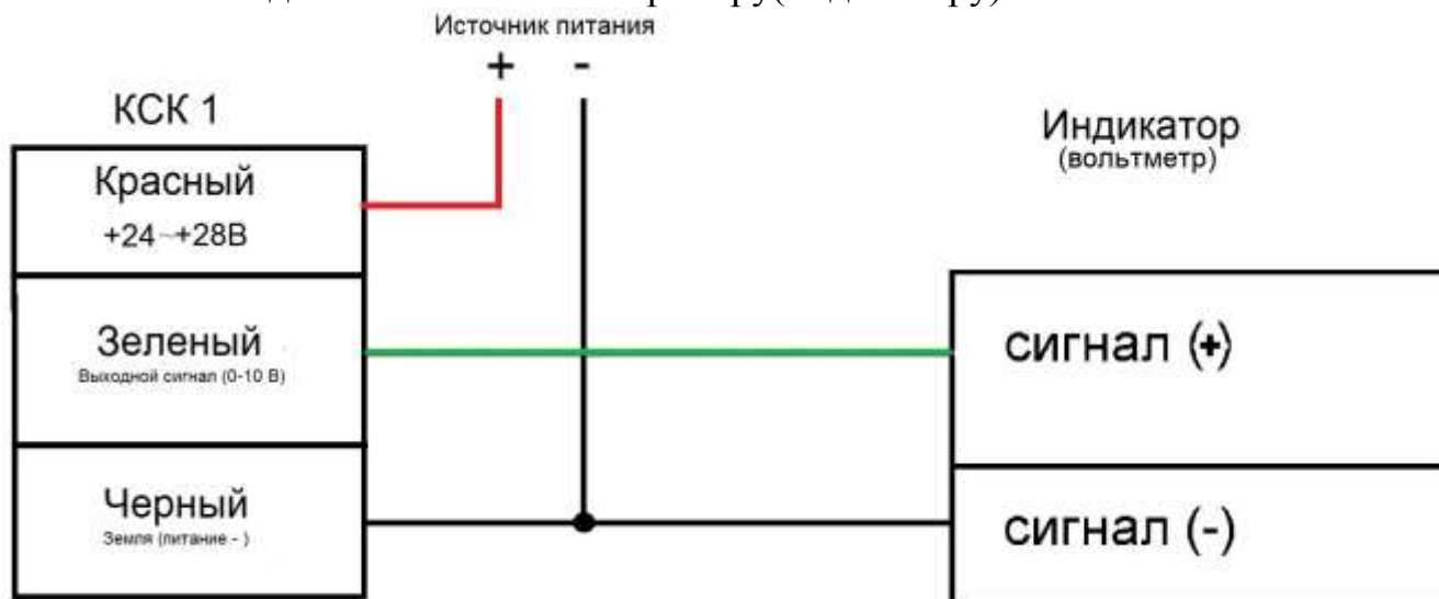
Рис1. Схема подключения КСК 1 к прибору(индикатору).
