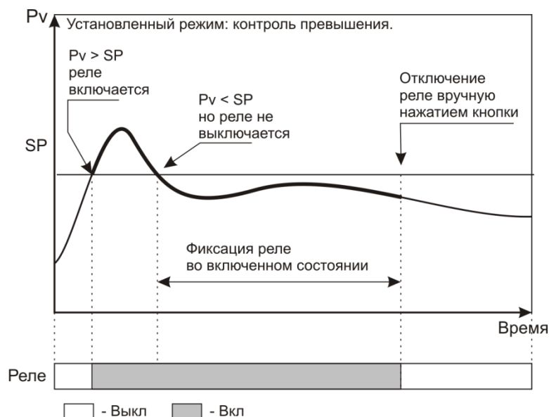
Рисунок.7 Иллюстрация работы прибора в режиме фиксации включения реле.
